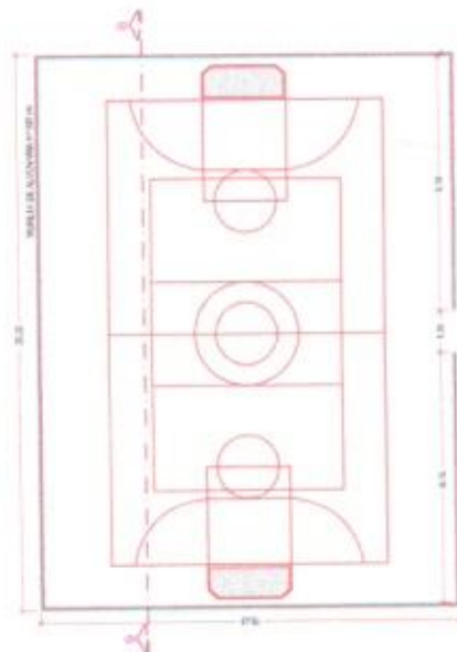
06 PLANTA BAIXA QUADRA Escala 1:50
