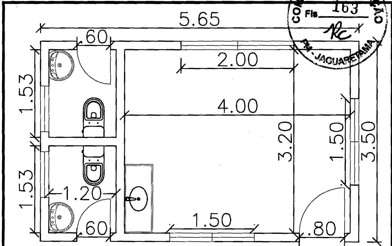
PLANTA BAIXA SEM ESCALA - METROS
