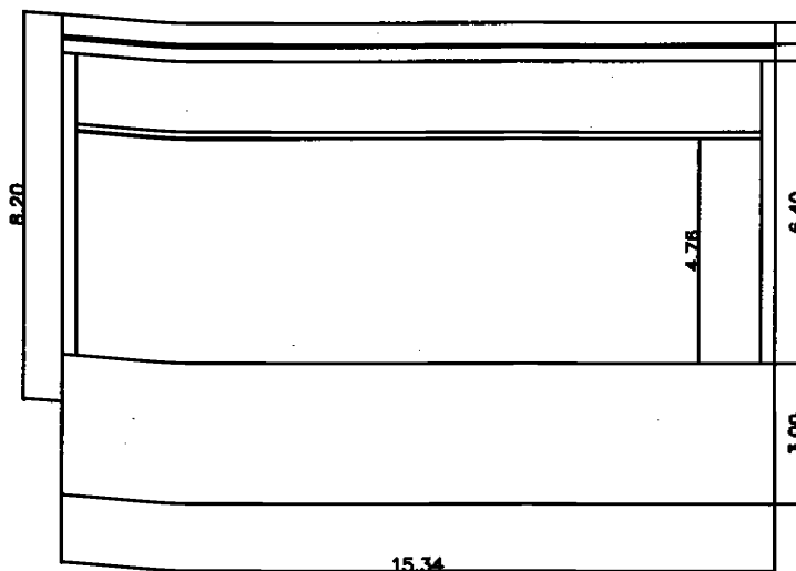
VISTA FRONTAL em 1/100
