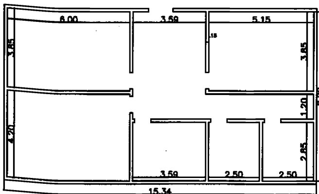
PLANTA BAIXA em 1/100
