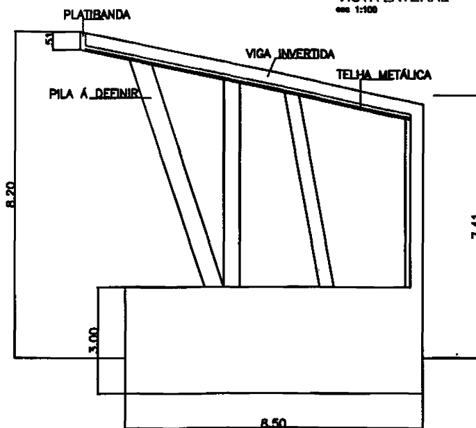
VISTA LATERAL esc 1:100
