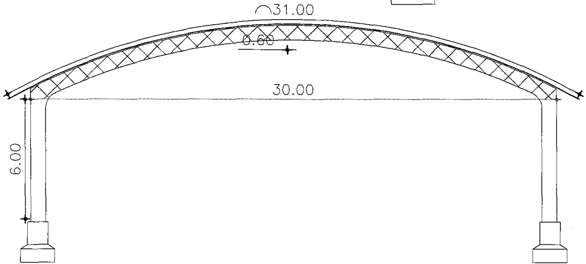
03 CORTE AA ESCALA _____ METROS
